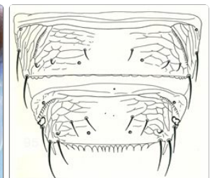
Tergites VII-VIII
