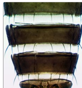
Sternites V-VII
