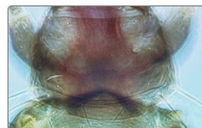
Pronotum
