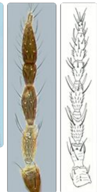
Antenna Antenna
