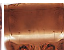
Sternite VII
